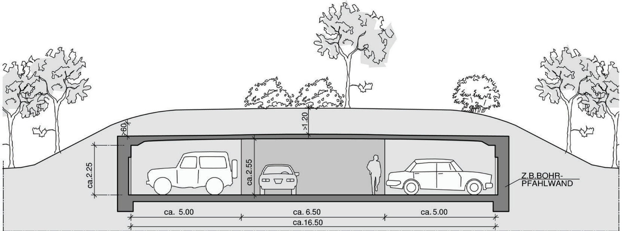
Skizze Querschnitt Vorschlag Variante 1, M.1:1000
